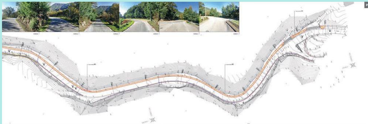
PLANTA PARCELAR - P2
